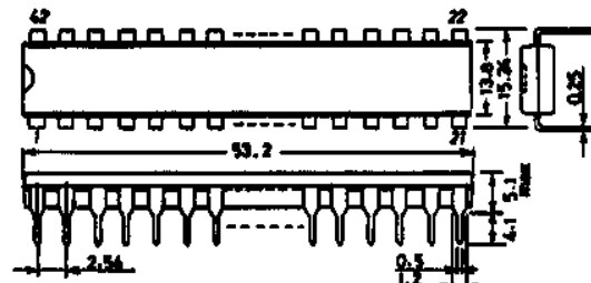
SANYO: DIP42
