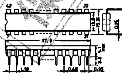
SANYO: DIP42S
